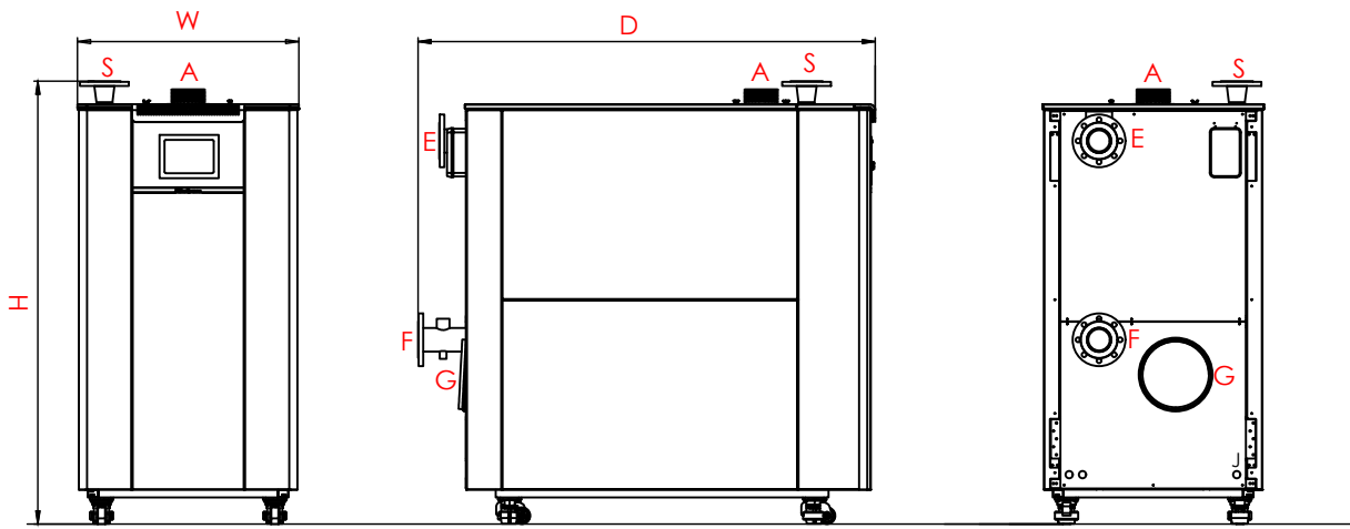
ALUBOX 540-700
