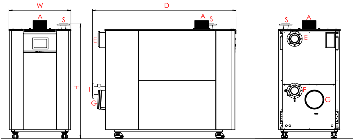
ALUBOX 1100
