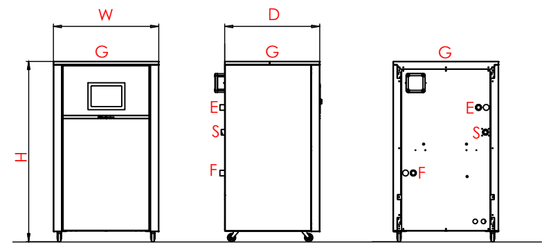
ALUBOX 540-700
