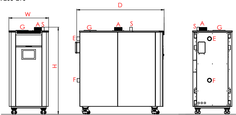
ALUBOX 208-290
